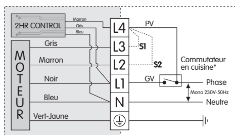
Schéma de câblage avec interrupteur
