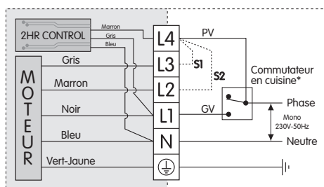
Schéma de câblage avec inverseur
