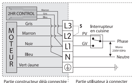
Schéma de câblage interrupteur va et vient
