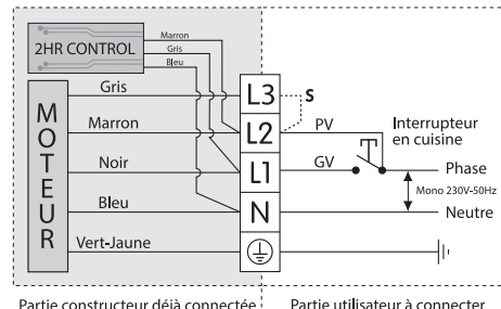
Schéma de câblage Bouton Poussoir
