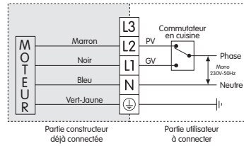
Schéma de câblage avec inverseur
