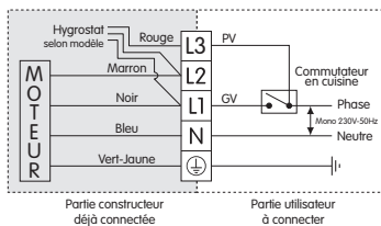
Schéma de câblage avec interrupteur
